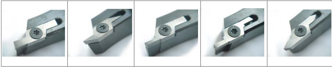
前挽き用 【INS-FR】 裏挽き用 【INS-BR】 突切り用 【INS-CR】 溝入れ用 【INS-GR】 ネジ切り用 【INS-SR】
